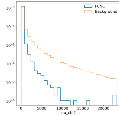
(f) \chi^2_{\nu}
