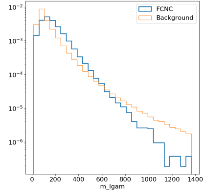
(d) m_{l\gamma}
