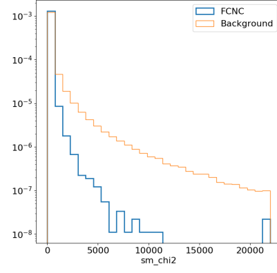
(d) \chi^2_{bW}
