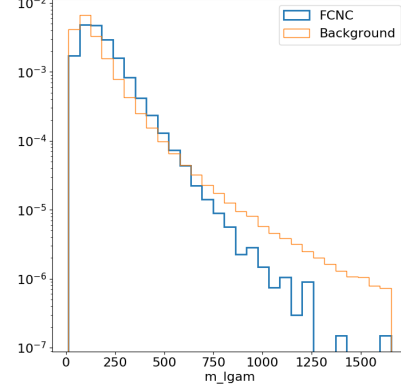
(d) m_{l\gamma}
