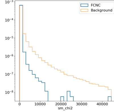
(d) \chi^2_{bW}
