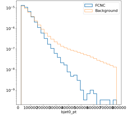
(d) p_T(b)
