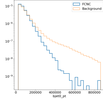
(d) p_T(b)
