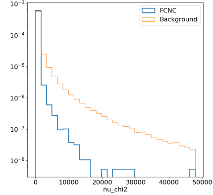
(f) \chi^2_\nu
