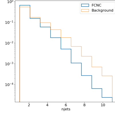
(d) n_{jets}
