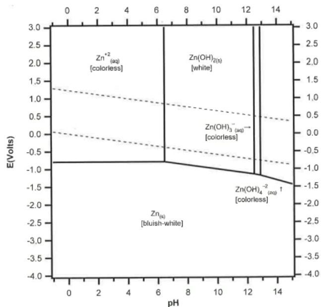
Figure 9. Pourbaix diagram for zinc. 20
